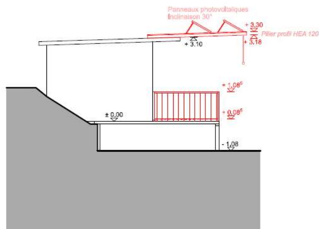
Façade Ouest
