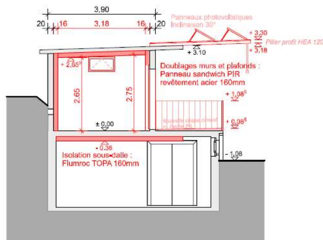
Coupe A-A
